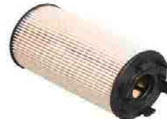
GE 3023 FPL Mercedes 9360903855 OD 74/62 ID1 32 ID2 30 H 161/140
