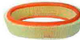
GA 0872 P Renault 7701047655 OD 264 ID1 200 ID2 200 H 89
